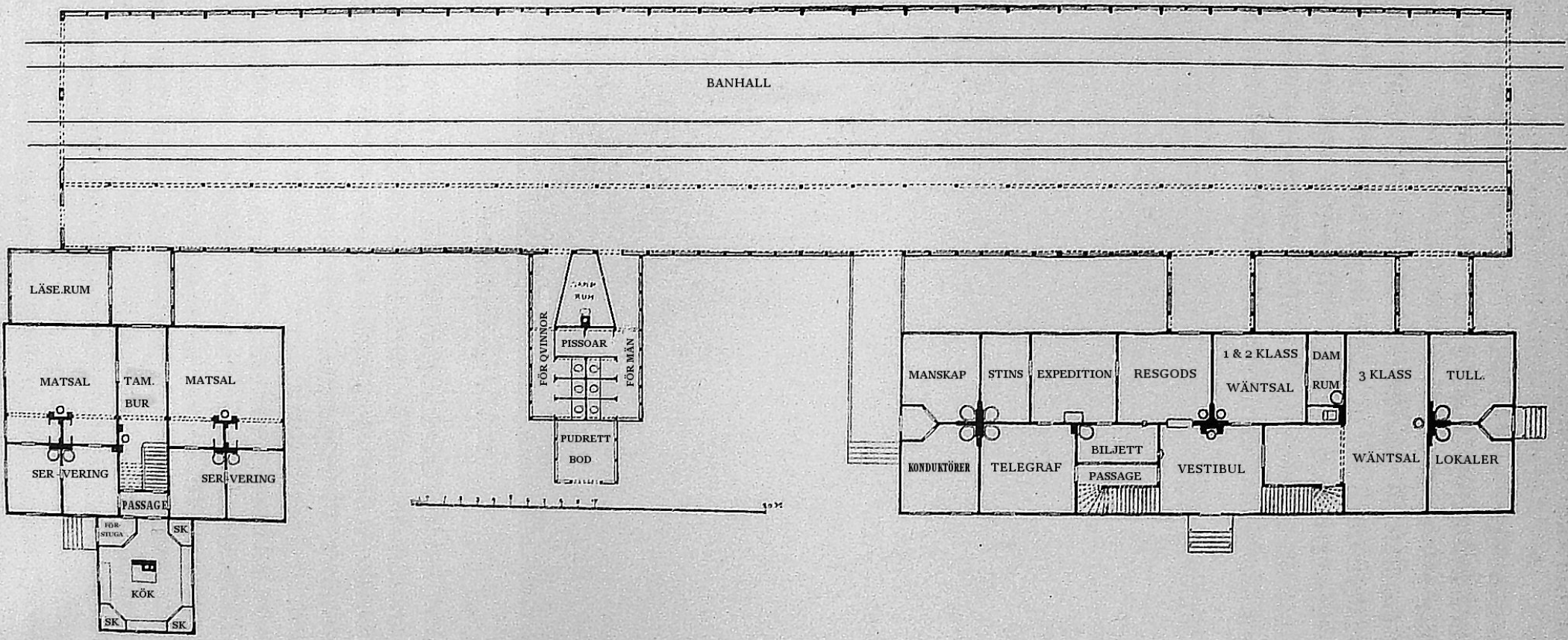
260. Plan af Storliens stationshus med banhall.
